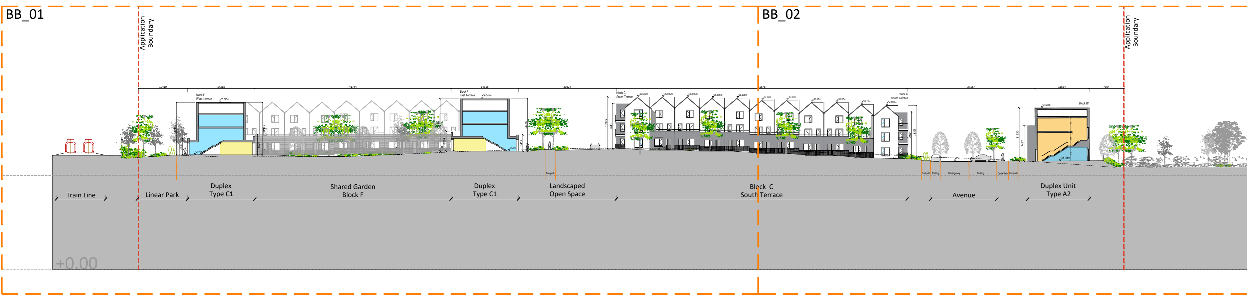
Section BB Esc 1:500
